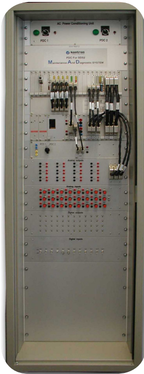
Bild 3: Das Instandhaltungs- und Diagnosesystem ermöglicht es den Betreibern, die Funktionalität aller SDS 2 Bauelemente zu überprüfen.
