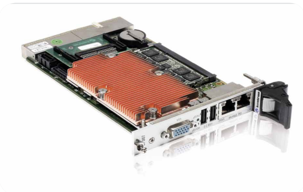
Bild 6: Das Herzstück der VESA- und VDEC-Einheiten: Kontrons CP307
